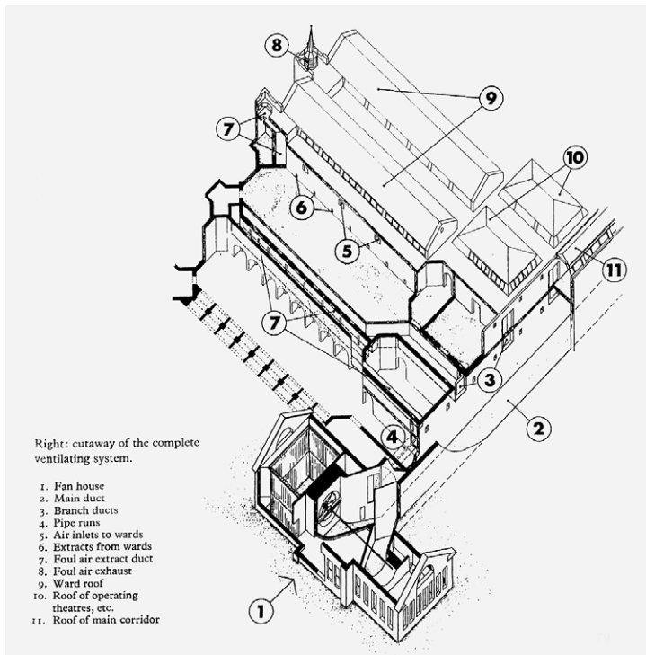
Abb. 6 Schnitt durch das Lüftungssystem des Royal Victoria Hospital in Belfast
