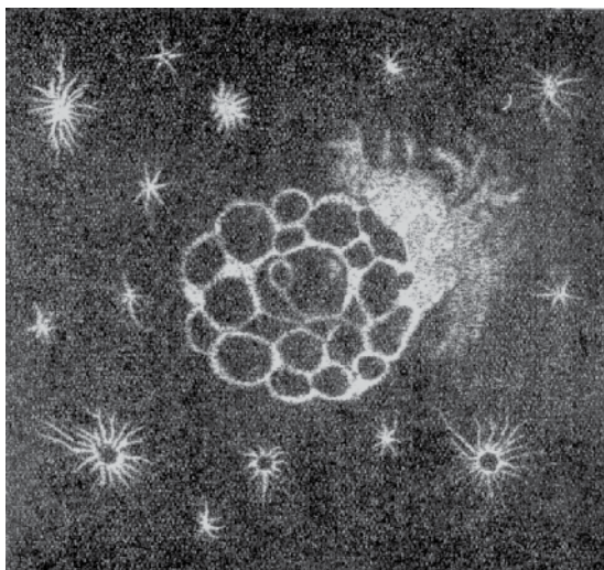
Abb.2: Lichtenberg-Figur
