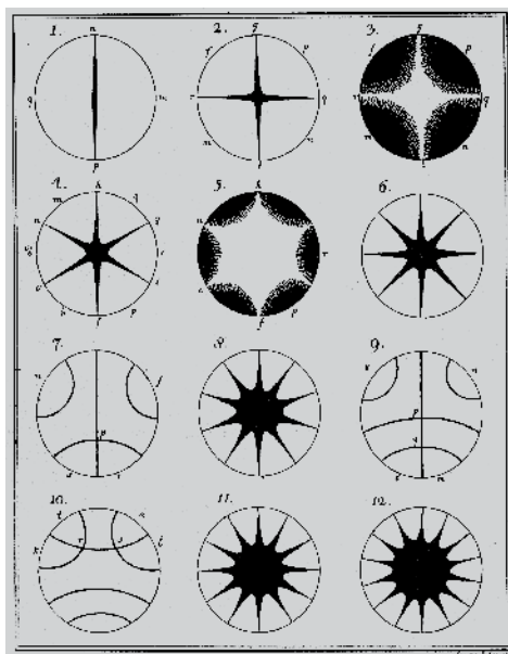
Abb. 9: Chladni: Klangfiguren
