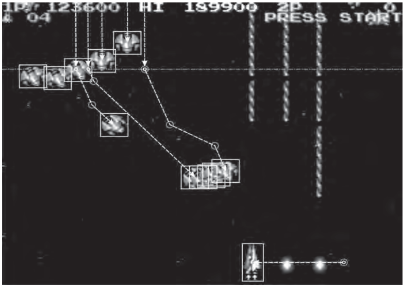
Abb. 4: Screenshot aus SALAMANDER (1986) mit beispielhaft eingezeichneten Trajektorien und Bounding Boxes. Die horizontale Linie stellt einen vertikalen Positionsgrenzwert dar, bei deren Überschreitung die Gegner ihre Patternsequenz wechseln.
