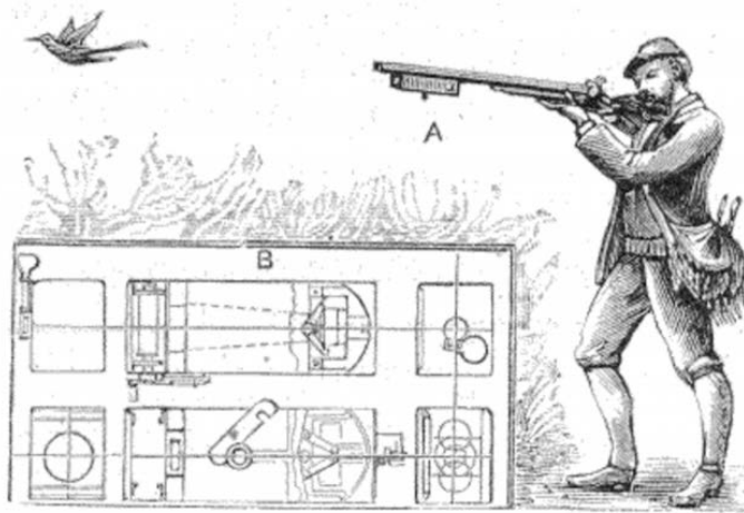
Le fusil photographique ou chambre noire du chasseur. A. Mode d'emploi de l'appareil. — B. Schéma du mécanisme.
