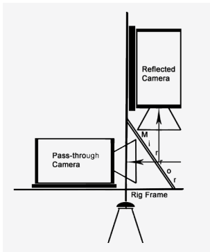
13 Beamsplitter rig.
